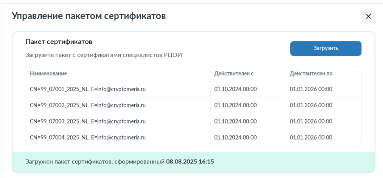
Рис. 3.18. Окно «Управление пакетом сертификатов». Просмотр содержимого пакета с сертификатами
